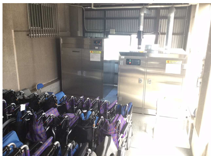
・マルチドライヤー(電気式多目的乾燥機) とトルネード(全自動車いす洗浄消毒機)
